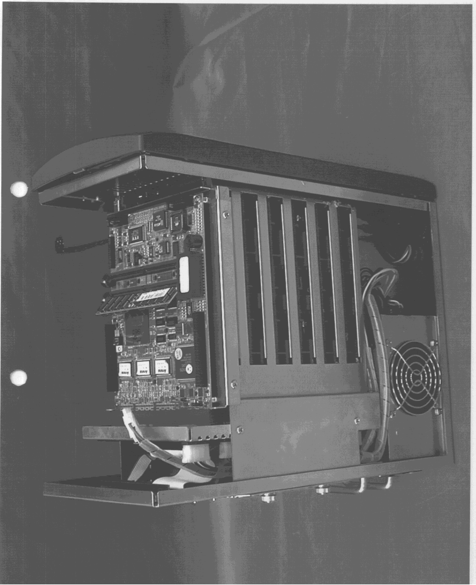
FCC ID : NKF-ARENA LE PHOTO 4. EUT INSIDE VIEW
