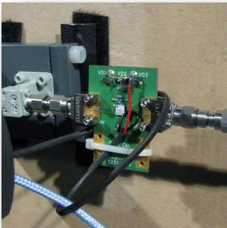
LNA
