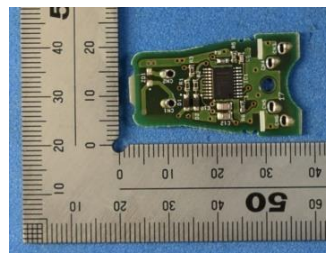
Bottom (PCB)
