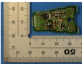
Top (PCB)
