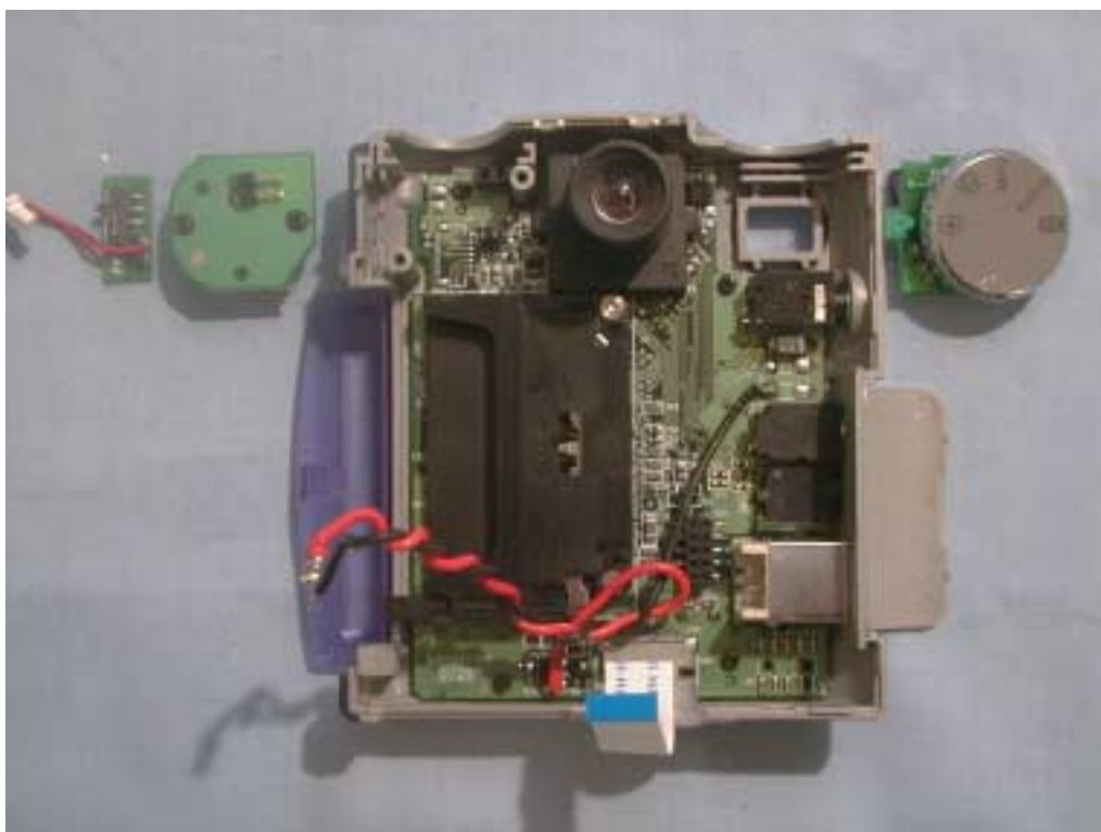
(12) EUT Photo
