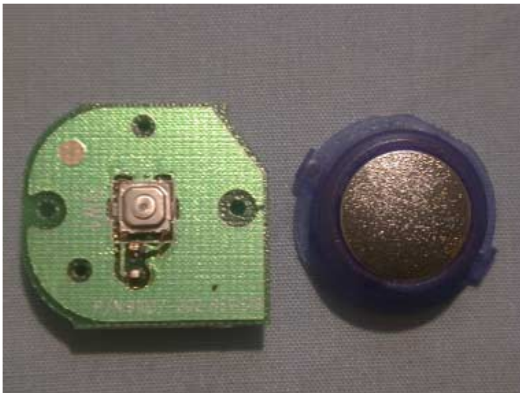
(14) EUT Photo
