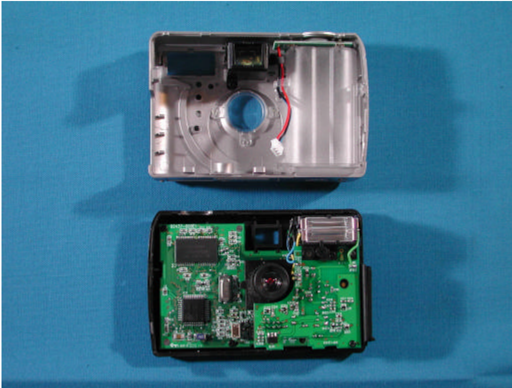
(6) EUT Photo
