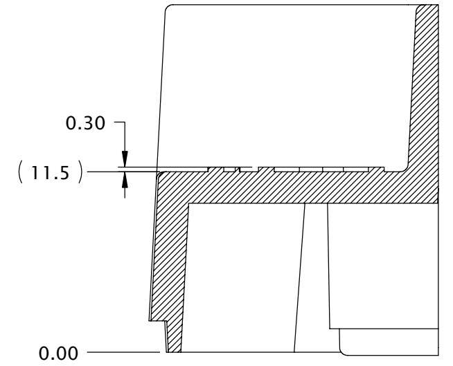
SECTION V-V SCALE 2 : 1
