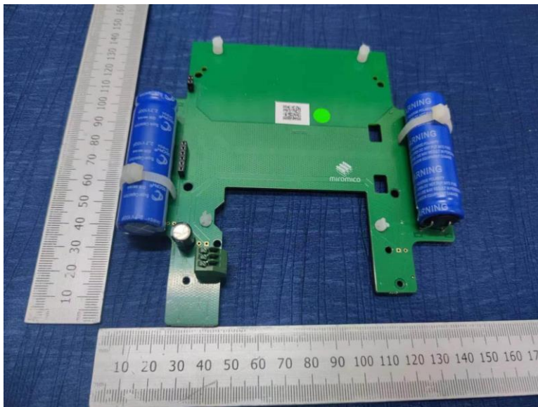
FLRC module
