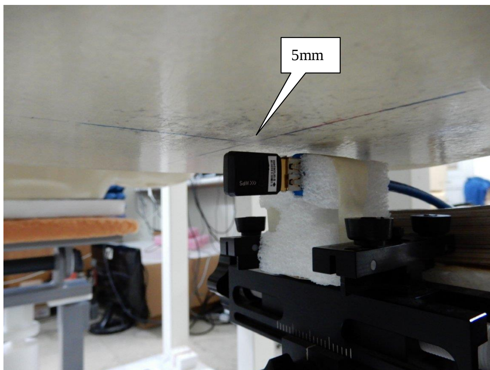
EUT Left-Side
