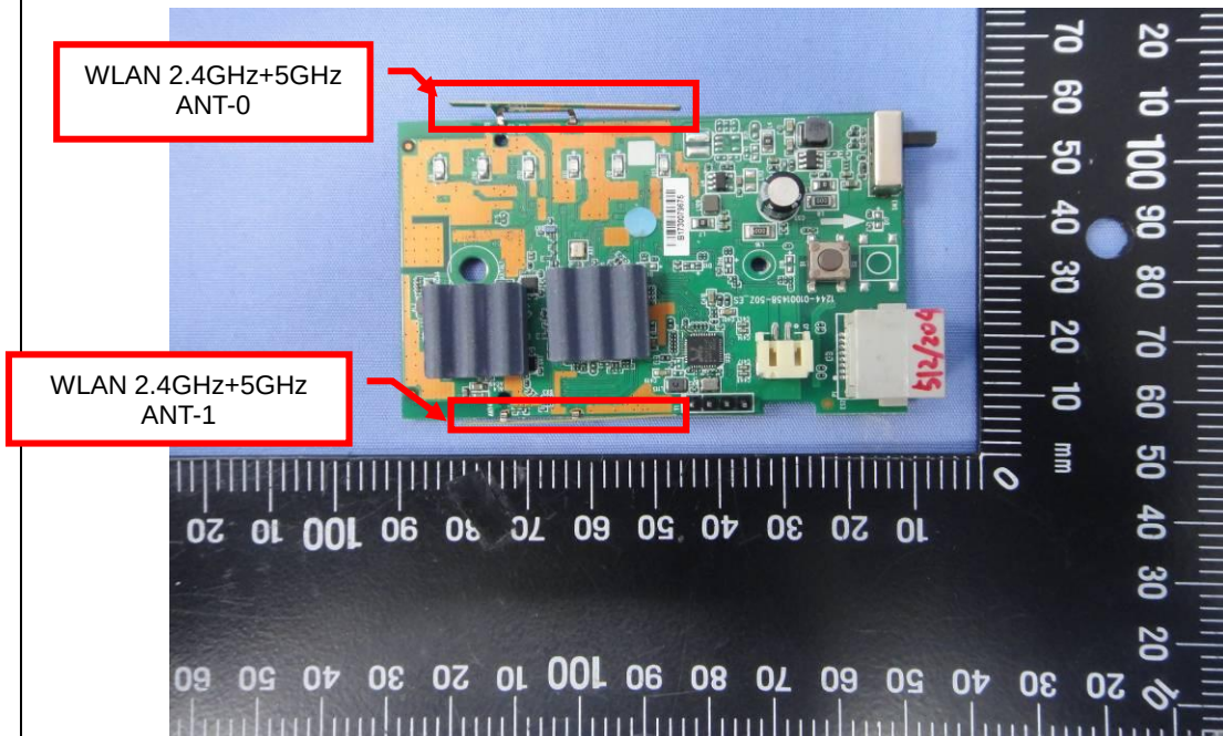
EUT Photo (2)
