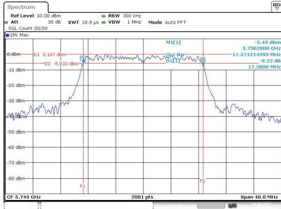
11N5.8G-20M – F1 [Port 1]
