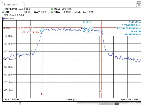
11N5.8G-20M – F2 [Port 1]
