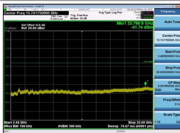
,Plot 4,2483.5MHz~25000MHz-802.11n(HT 20),2462MHz,Ant0
