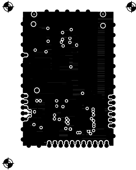
SOLD. LAYER
