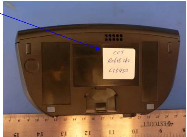
Base (EUT)
