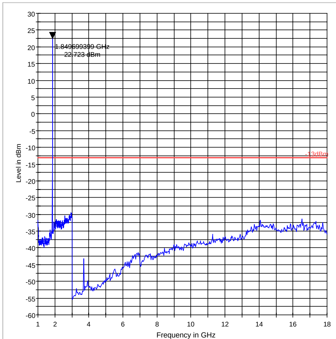
FCC 24 1-18GHz
