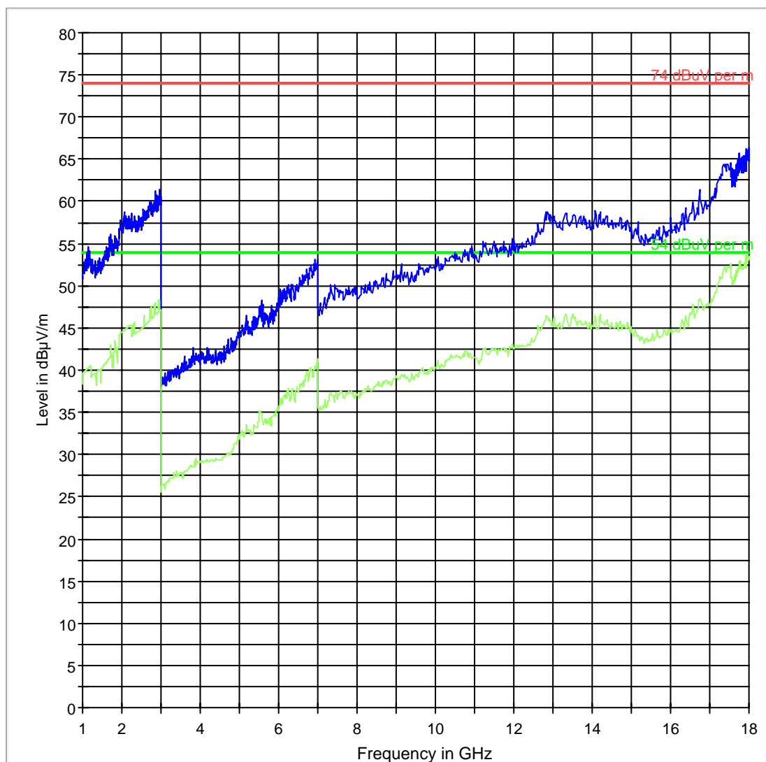
FCC 15 1-18GHz
