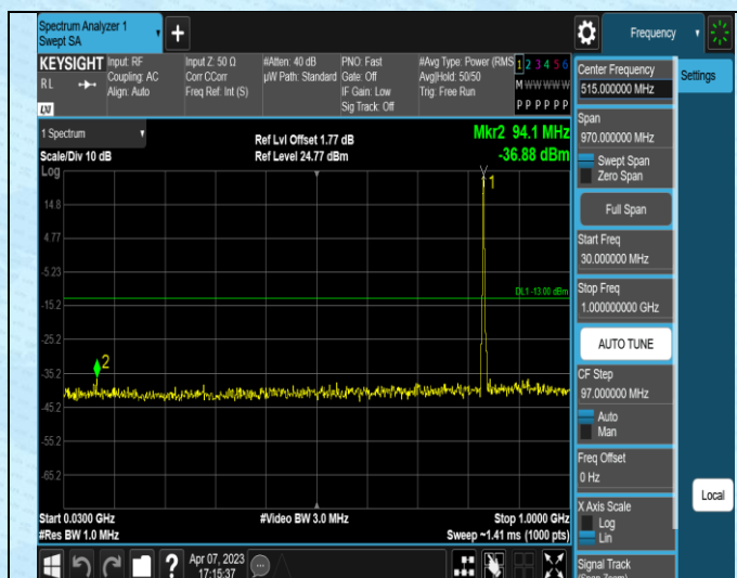
Band5-3MHz-QPSK-20635-1RB#0-Range2:30~1000MH
