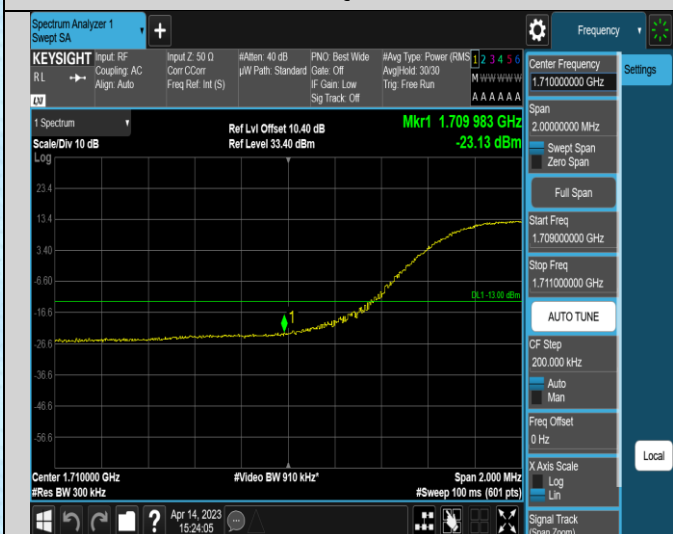
Band4-20MHz-QPSK-20050-100RB#0
