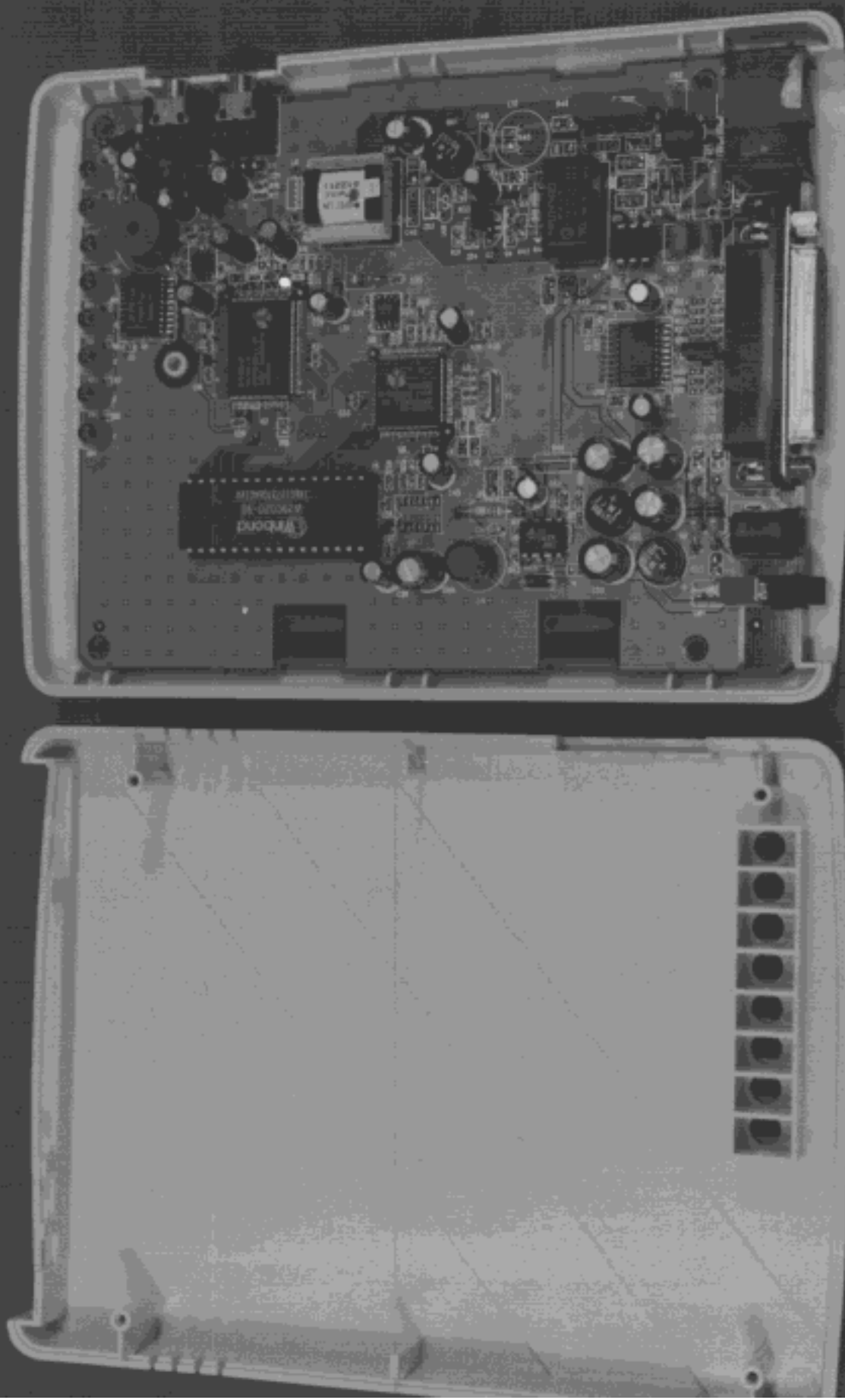
FCC ID : NBUF560XD-001 PHOTO 3. EUT INSIDE VIEW
