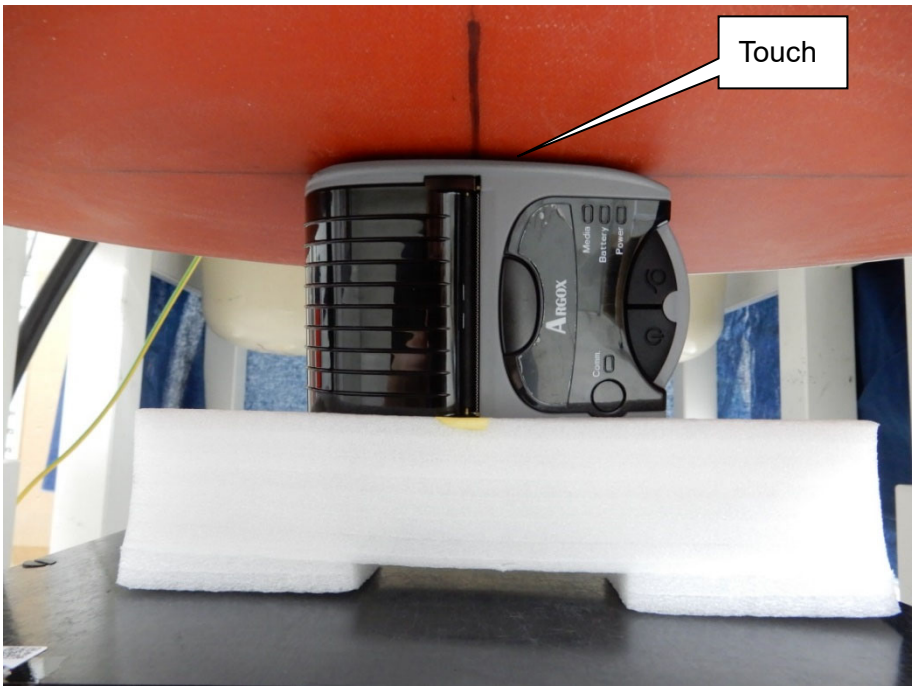
EUT Right-side
