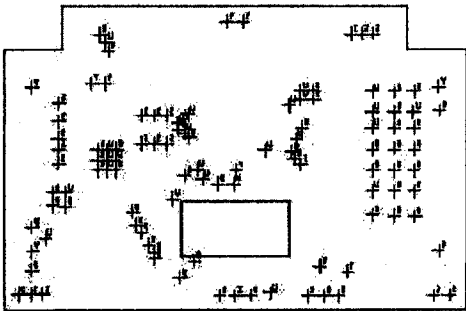
900-TPX301-10300V0 Silkscreen Top
