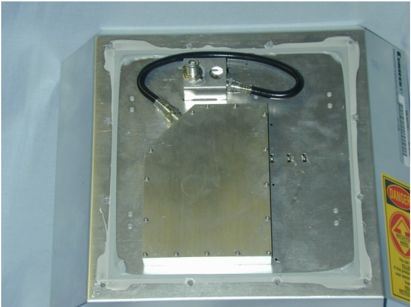
Photo 5 - Antenna Module
