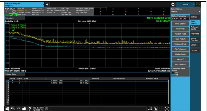
802.11a 5320M
