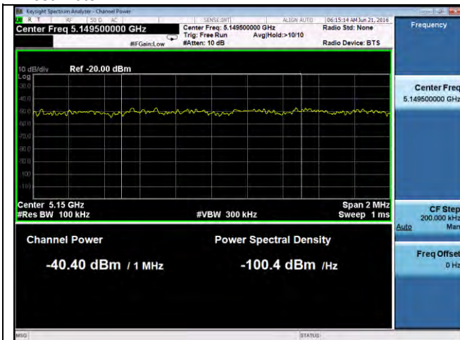
Band Edge -802.11a-5180M
