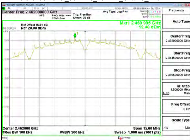
Reference Level 802.11b 20MHz Chain0 2462MHz
