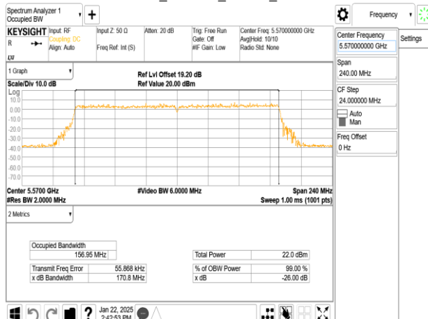
802.11be_160MHz_Chain1_5570MHz
