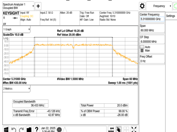
802.11n_40MHz_Chain1_5310MHz
