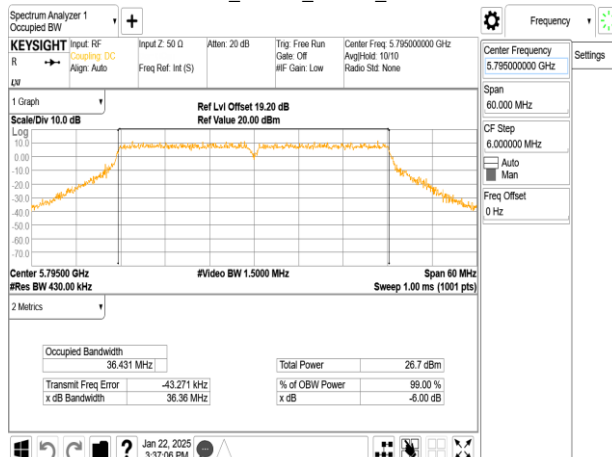
802.11n_40MHz_Chain1_5795MHz
