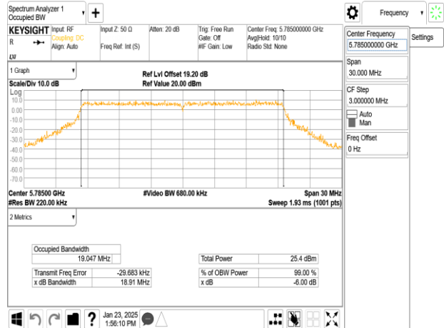
802.11be_20MHz_Chain0_5785MHz
