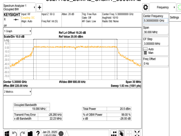
802.11be_20MHz_Chain1_5300MHz
