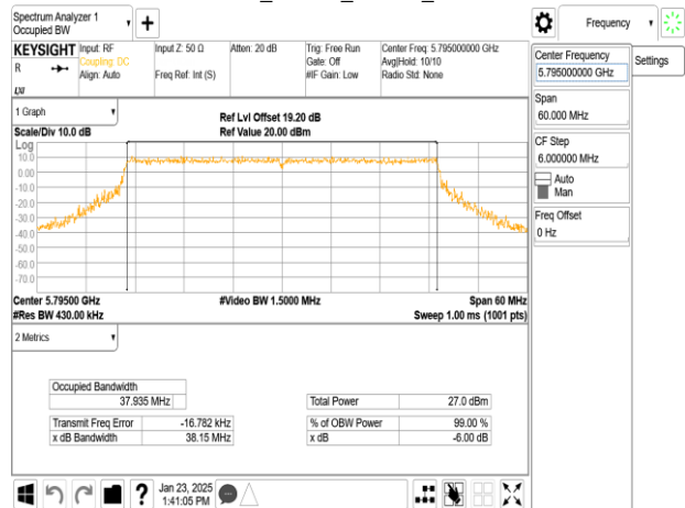
802.11be_40MHz_Chain0_5795MHz
