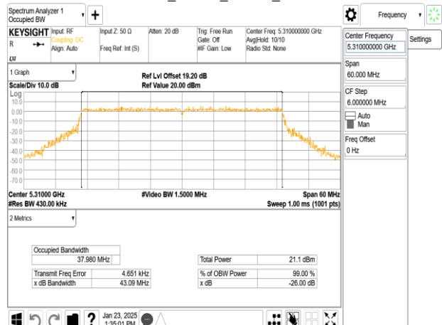
802.11be_40MHz_Chain0_5310MHz
