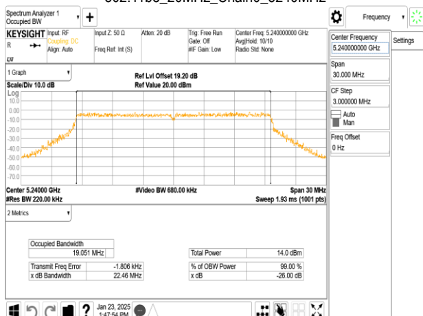
802.11be_20MHz_Chain0_5240MHz
