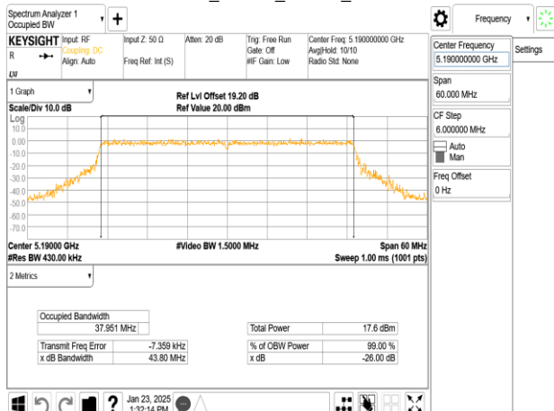
802.11be_40MHz_Chain0_5190MHz
