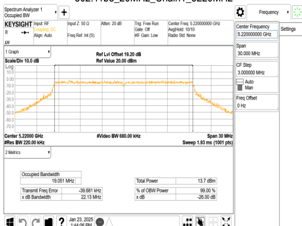
802.11be_20MHz_Chain1_5220MHz
