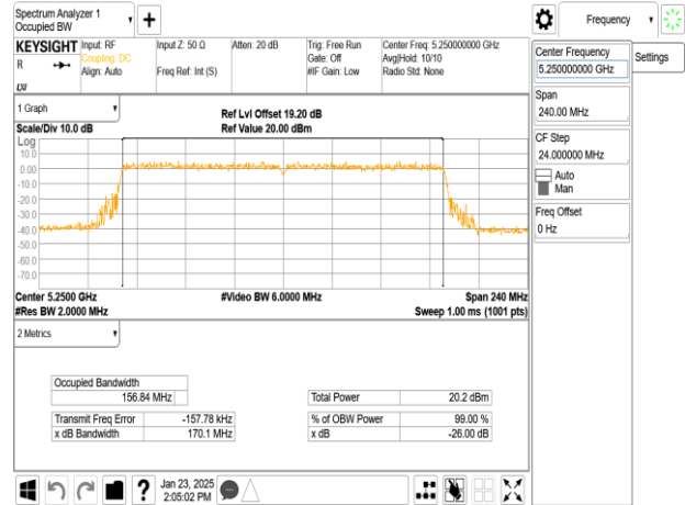
802.11be_160MHz_Chain1_5250MHz
