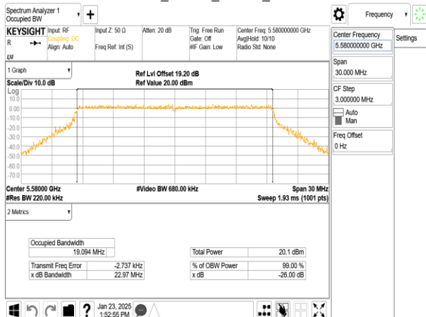
802.11be_20MHz_Chain1_5580MHz
