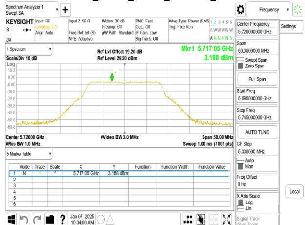
802.11a_20MHz_Chain0_5720MHz_UNII 3
