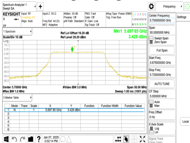
802.11be_20MHz_Chain0_5700MHz
