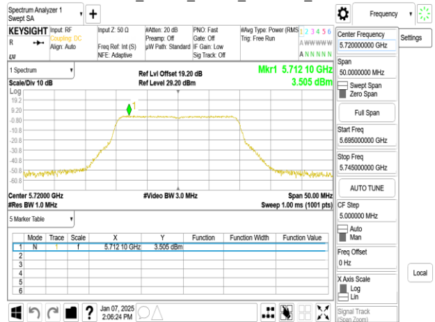
802.11be_20MHz_Chain0_5720MHz_UNII 3
