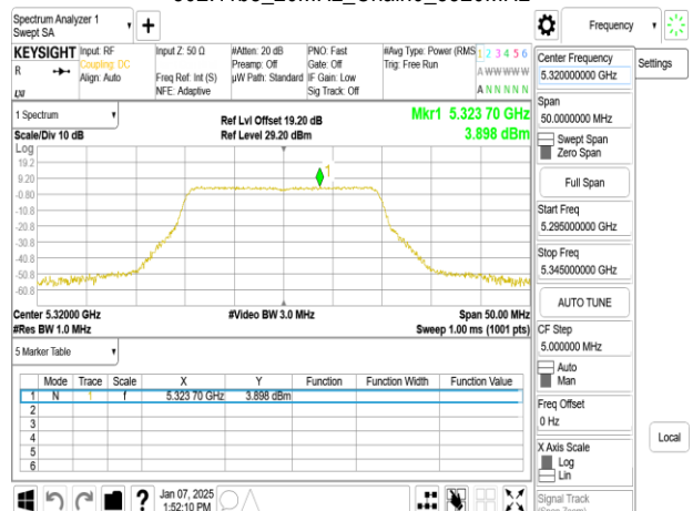
802.11be_20MHz_Chain0_5320MHz
