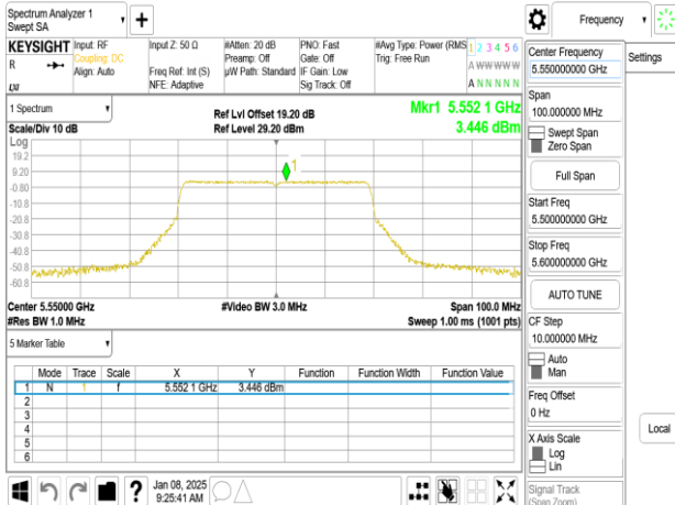
802.11be_40MHz_Chain1_5550MHz
