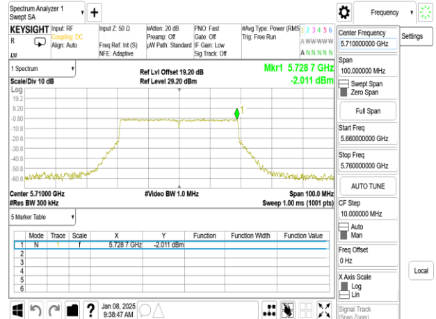
802.11be_40MHz_Chain1_5710MHz_UNII 3
