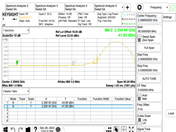
802.11b_20MHz_Chain1_2417MHz
