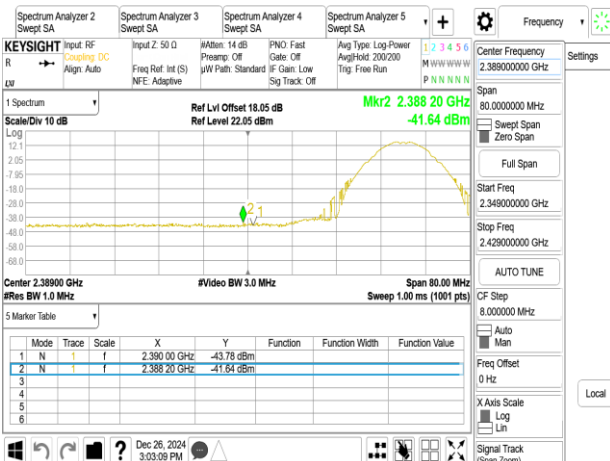
802.11b_20MHz_Chain0_2422MHz
