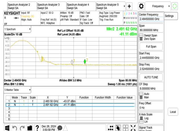
802.11b_20MHz_Chain0_2457MHz
