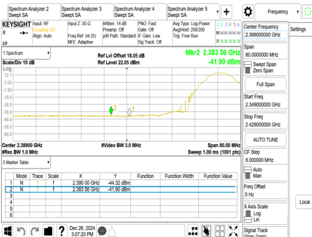
802.11b_20MHz_Chain0_2422MHz
