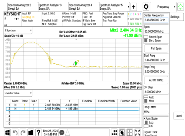
802.11b_20MHz_Chain0_2457MHz
