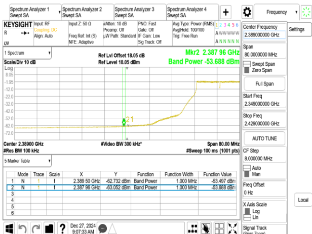
802.11g_20MHz_Chain1_2427MHz
