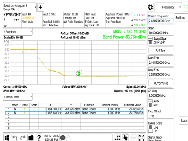
802.11g_20MHz_Chain1_2457MHz
