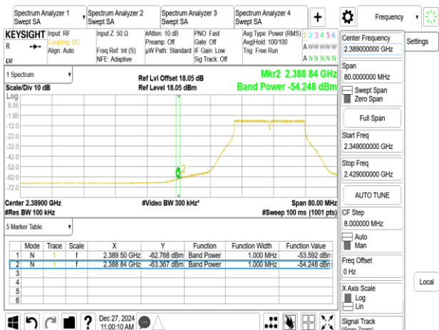
802.11n_20MHz_Chain0_2417MHz
