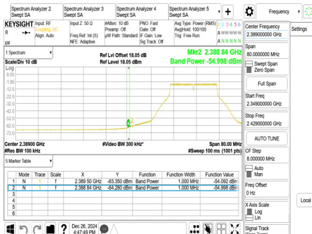
802.11g_20MHz_Chain1_2417MHz
