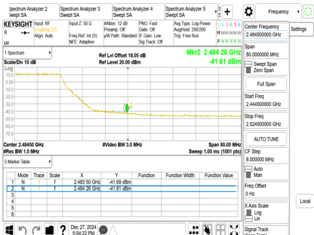
802.11be_40MHz_Chain1_2447MHz
