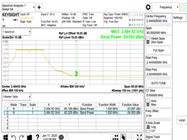
802.11g_20MHz_Chain0_2457MHz
