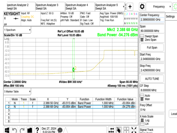
802.11be_40MHz_Chain1_2432MHz
