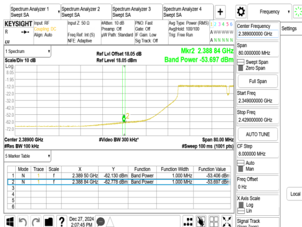
802.11n_40MHz_Chain0_2432MHz
