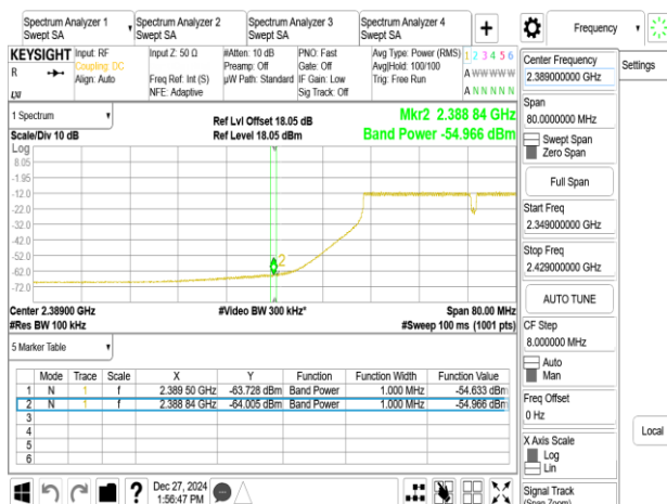
802.11n_40MHz_Chain1_2427MHz
