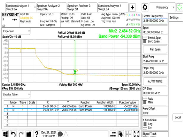
802.11n_20MHz_Chain0_2457MHz
