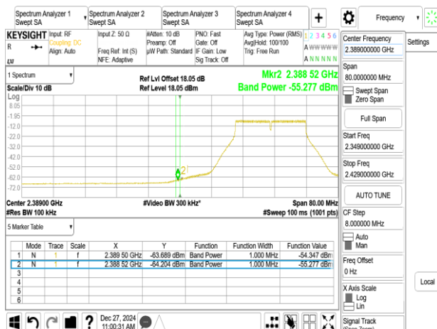
802.11n_20MHz_Chain1_2417MHz
