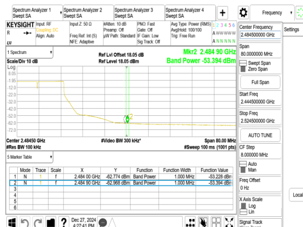
802.11be_20MHz_Chain1_2452MHz
