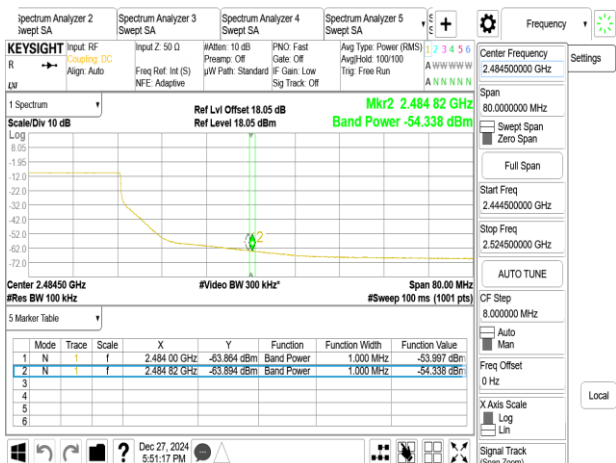
802.11be_40MHz_Chain0_2447MHz
