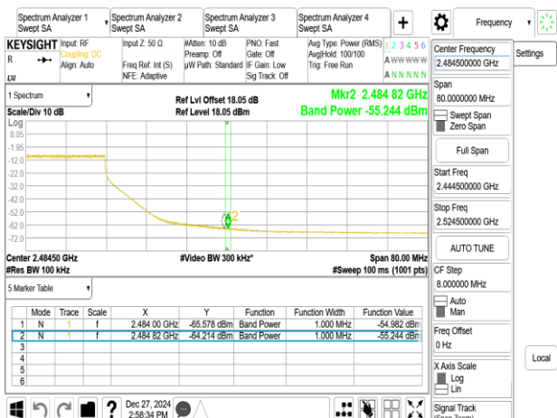
802.11n_40MHz_Chain1_2447MHz
