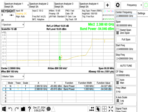
802.11be_20MHz_Chain0_2427MHz
