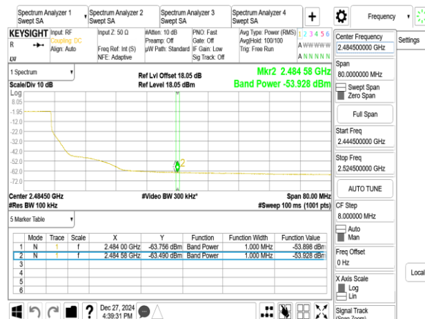
802.11be_20MHz_Chain1_2447MHz
