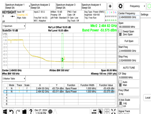
802.11n_20MHz_Chain1_2452MHz
