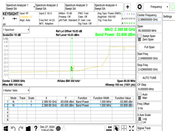
802.11be_20MHz_Chain1_2422MHz
