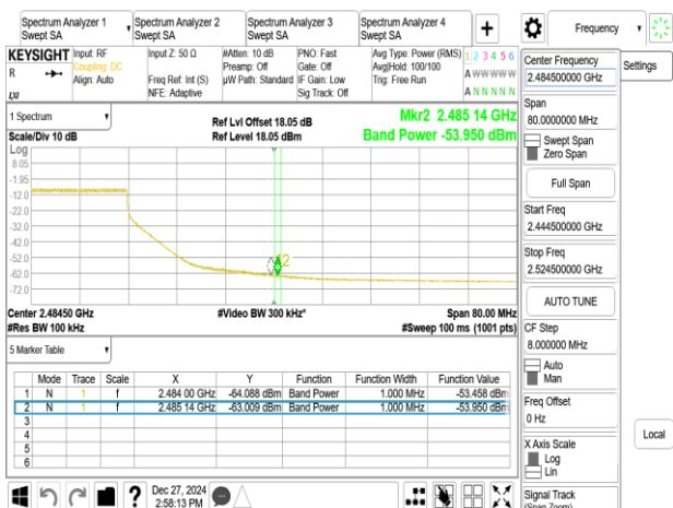
802.11n_40MHz_Chain0_2447MHz
