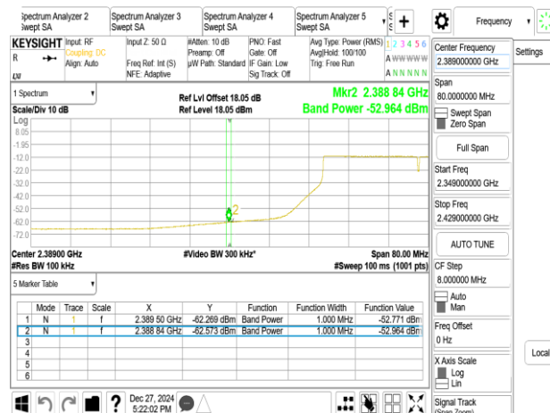
802.11be_40MHz_Chain0_2432MHz
