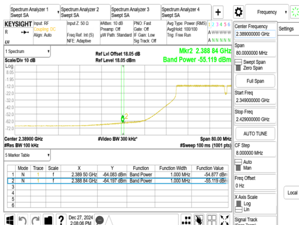
802.11n_40MHz_Chain1_2432MHz
