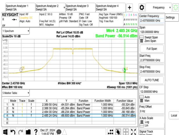
802.11n_40MHz_Chain1_2442MHz
