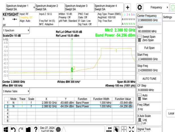
802.11be_20MHz_Chain0_2417MHz
