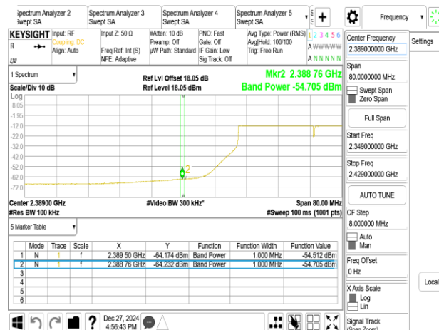
802.11be_40MHz_Chain1_2427MHz
