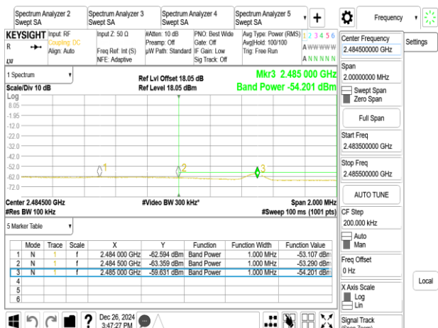
802.11b_20MHz_Chain1_2457MHz
