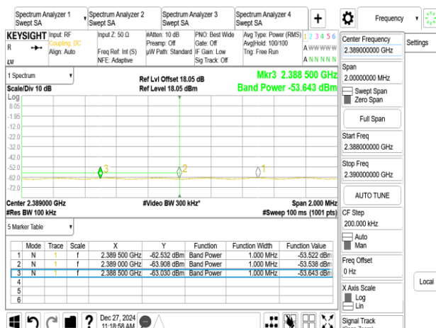
802.11n_20MHz_Chain1_2422MHz
