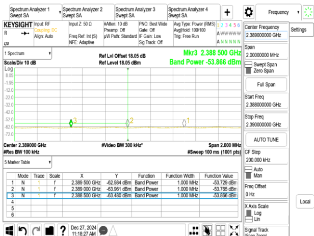
802.11n_20MHz_Chain0_2427MHz
