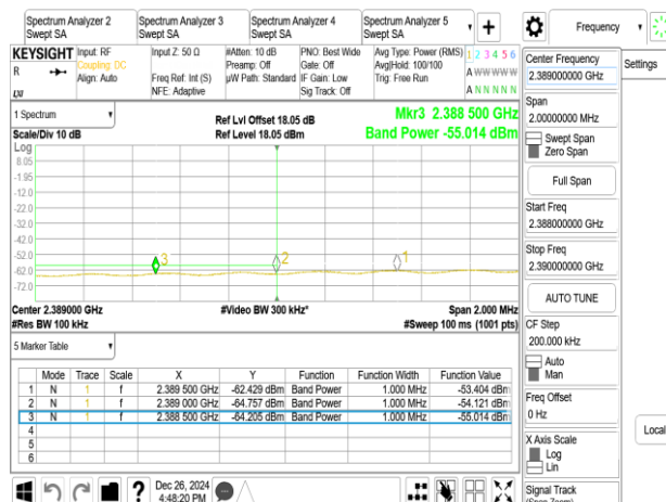
802.11g_20MHz_Chain0_2417MHz
