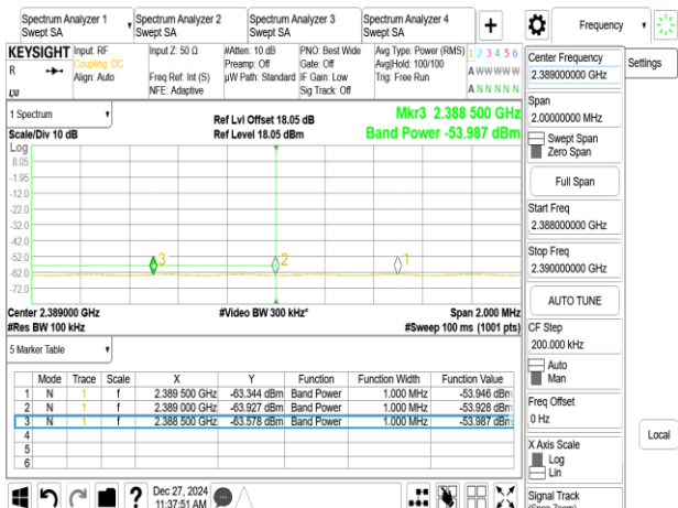
802.11n_20MHz_Chain1_2437MHz_L
