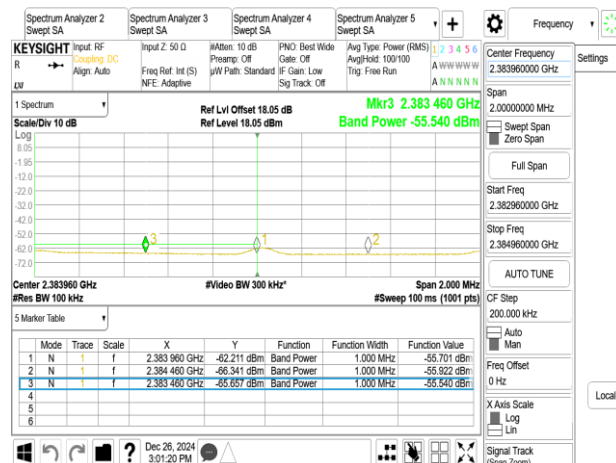
802.11b_20MHz_Chain1_2422MHz
