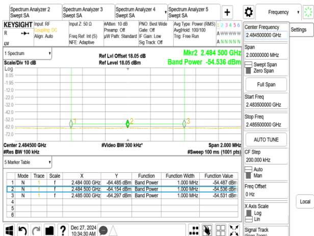
802.11g_20MHz_Chain1_2452MHz
