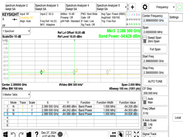
802.11be_40MHz_Chain1_2422MHz
