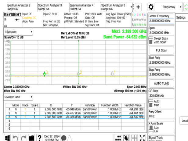
802.11be_40MHz_Chain1_2437MHz_L
