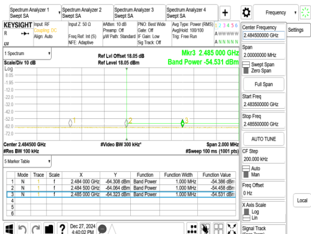
802.11be_20MHz_Chain0_2447MHz
