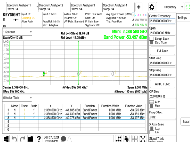
802.11n_40MHz_Chain0_2437MHz_L
