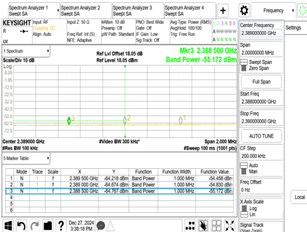
802.11be_20MHz_Chain1_2417MHz
