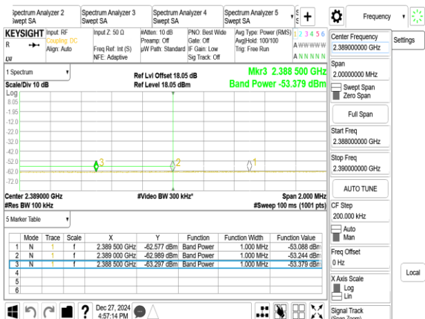
802.11be_40MHz_Chain0_2427MHz
