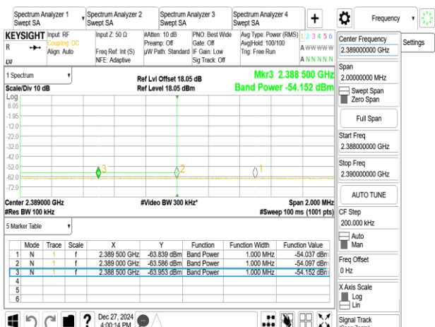
802.11be_20MHz_Chain0_2422MHz
