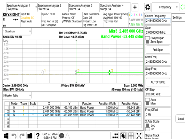
802.11be_20MHz_Chain1_2457MHz
