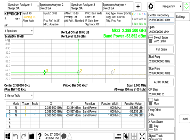
802.11be_20MHz_Chain1_2432MHz
