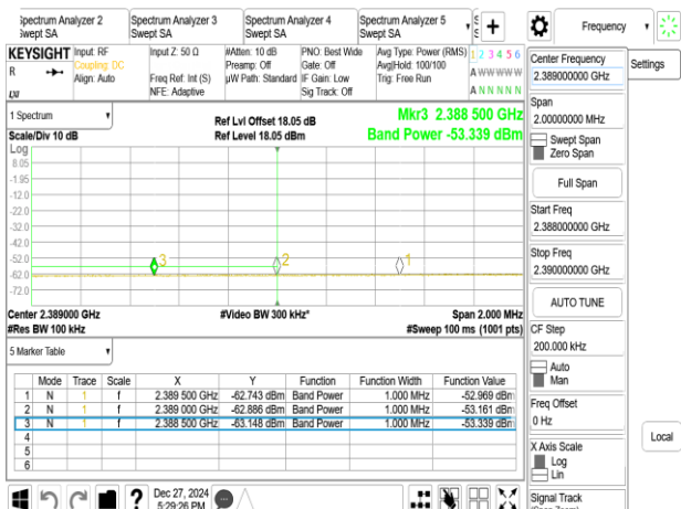
802.11be_40MHz_Chain0_2432MHz
