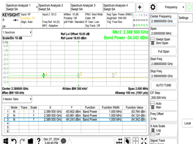
802.11be_20MHz_Chain0_2422MHz
