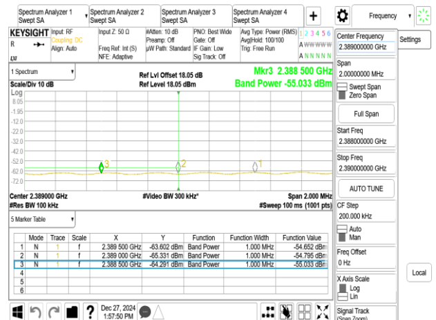
802.11n_40MHz_Chain1_2427MHz
