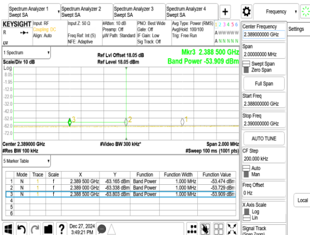
802.11be_20MHz_Chain1_2422MHz
