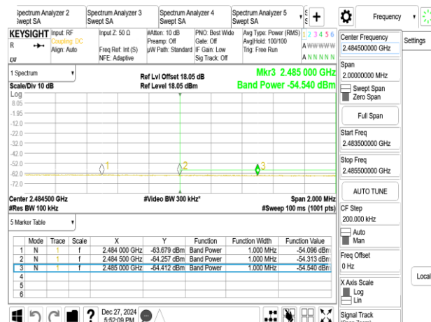
802.11be_40MHz_Chain0_2442MHz
