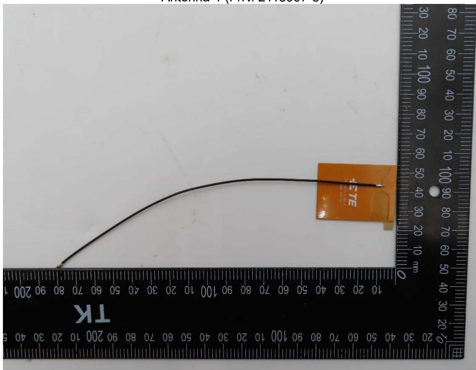
Antenna-1 (P/N: 2118907-8)
