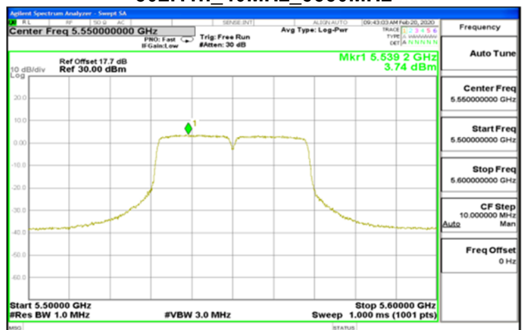
802.11n_40MHz_5550MHz
