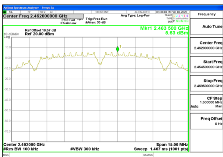
Reference Level_802.11b_20MHz_Chain2_2462MHz
