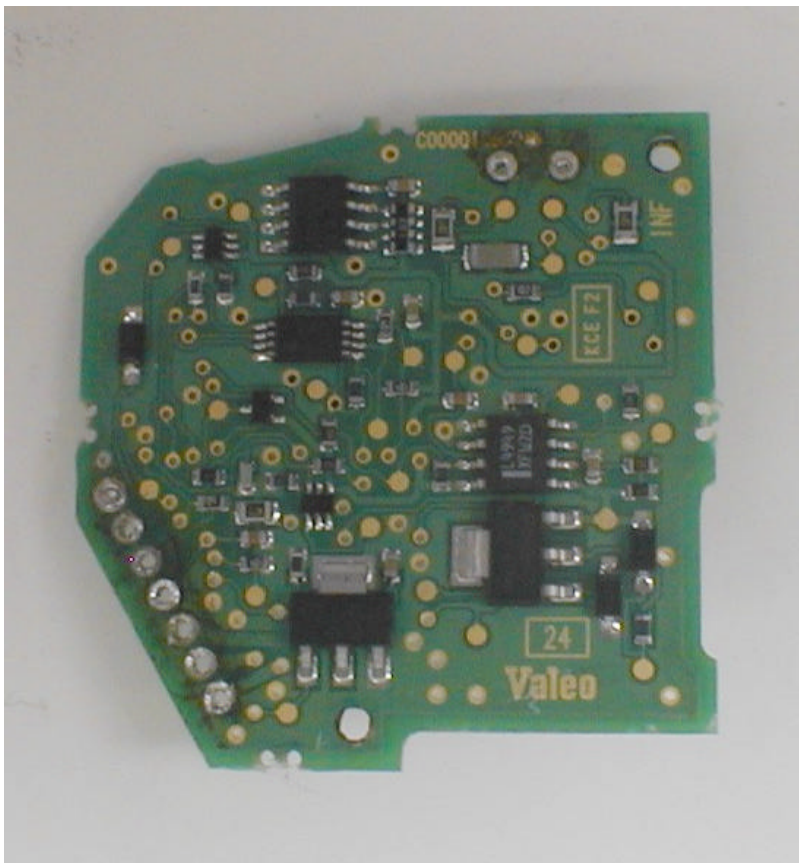
PCB Bottom
