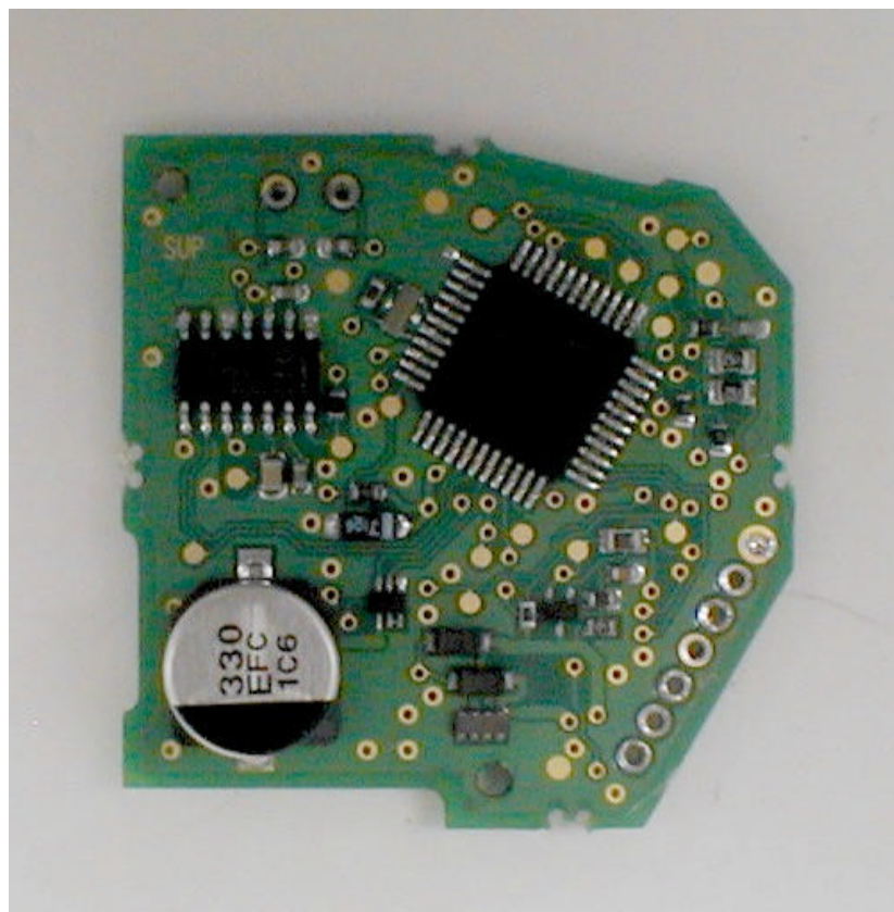
PCB Bottom
