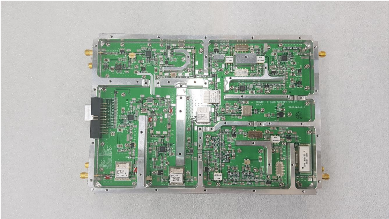
[SDR-7F RVS UDC MODULE]
