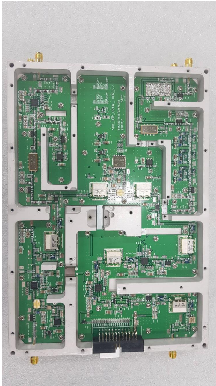
[SDR-CELL FWD UDC MODULE]
