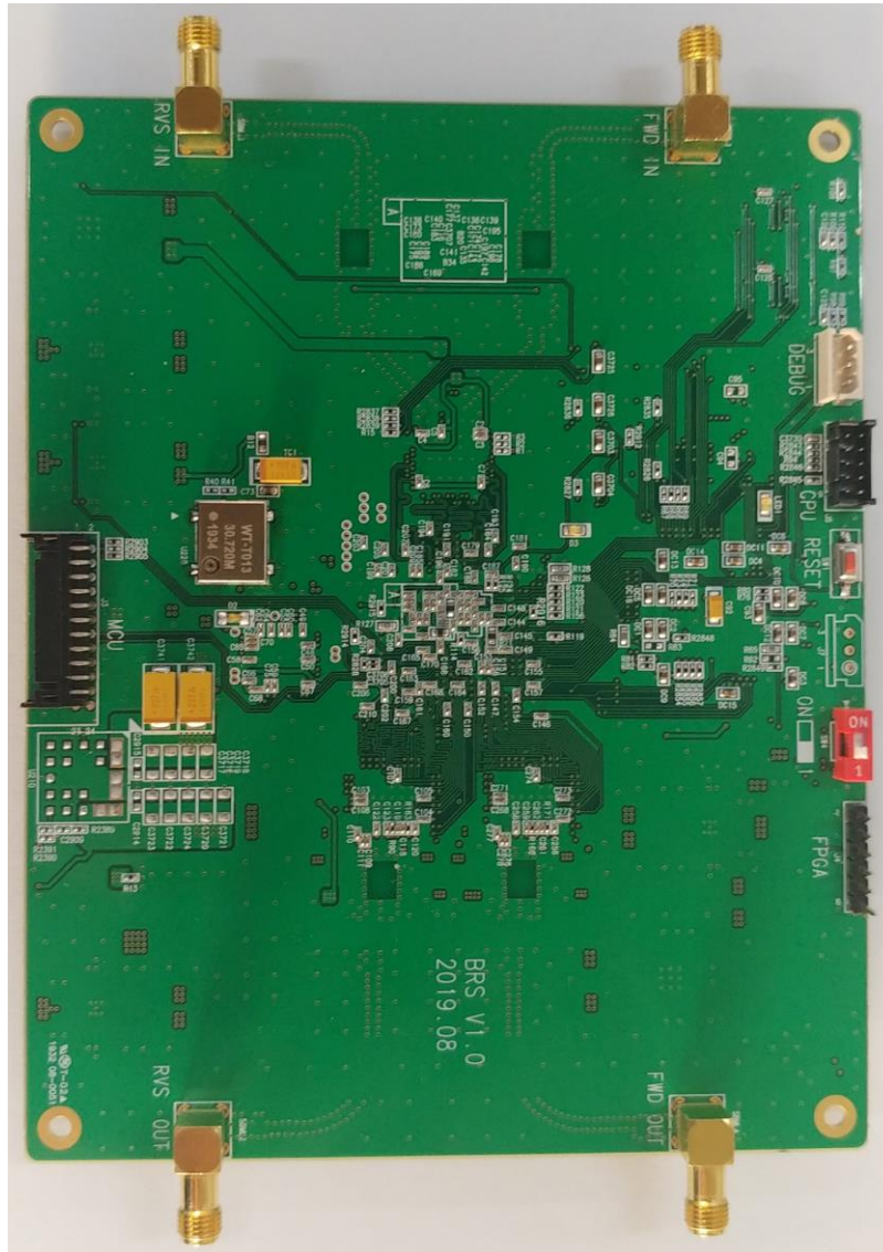
[DSP_4]
