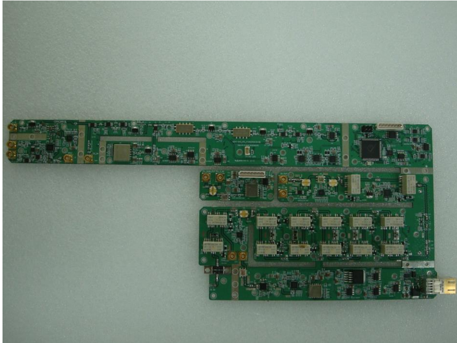
PBA TOP
