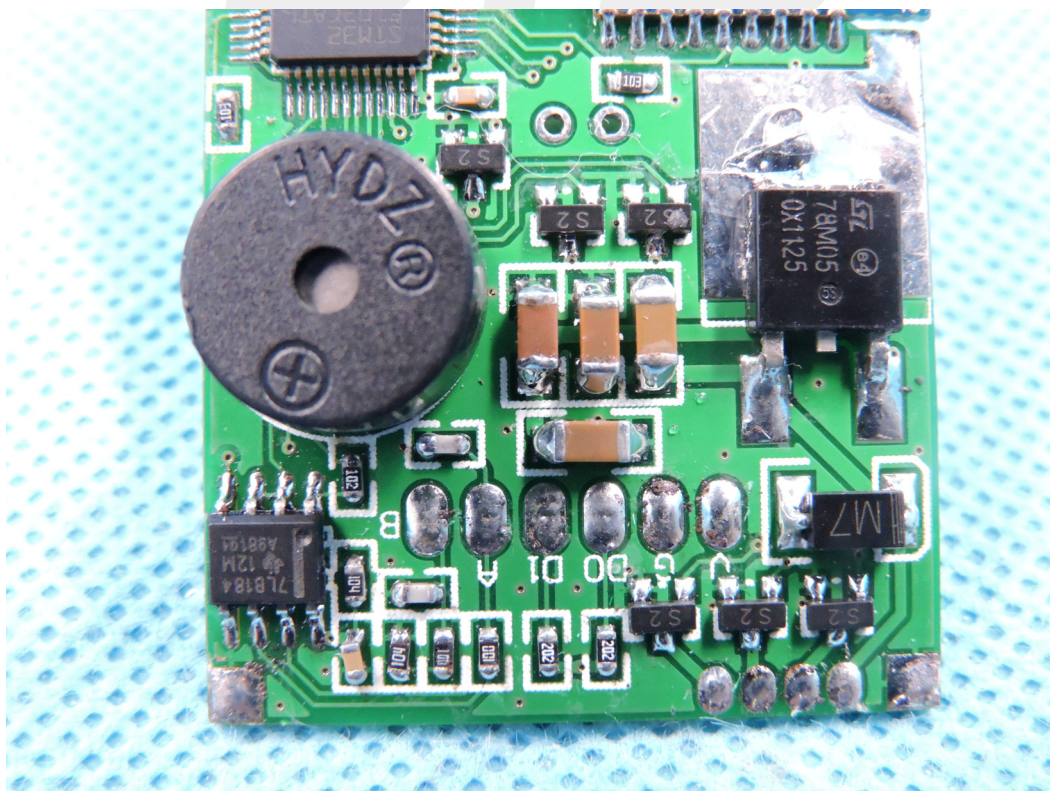
Photo 4 ( NXT-5M-KPD)
