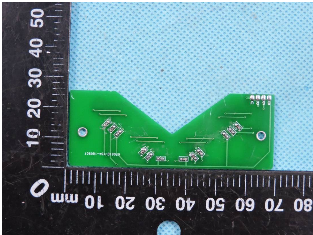
Photo 11 ( NXT-5M-KPD)
