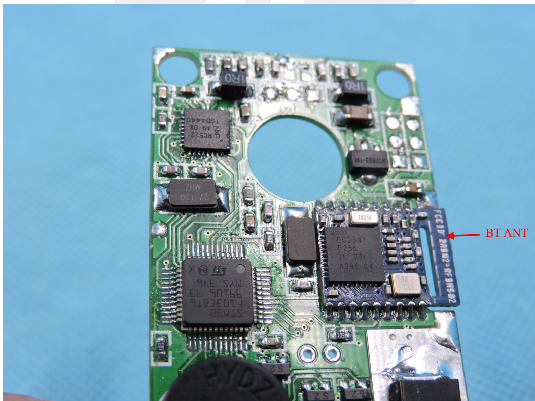
Photo 2 ( NXT-5M-KPD)
