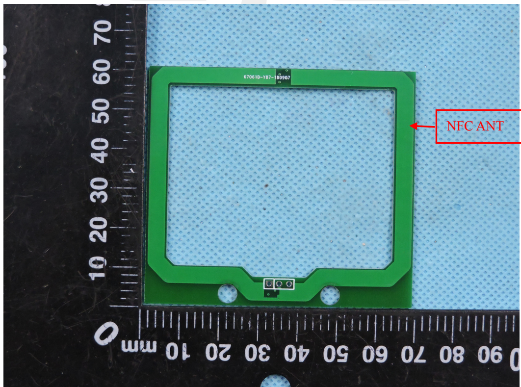
Photo 8 ( NXT-5M-KPD)
