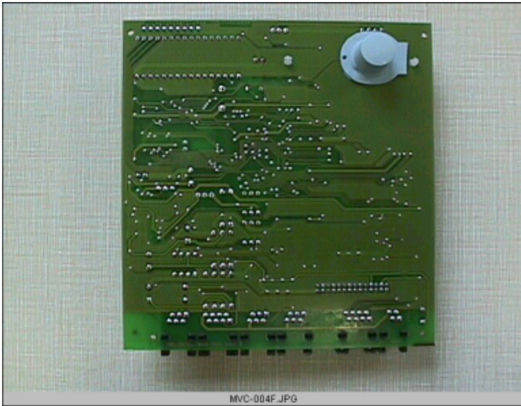
GPT Modem - Close Up of VIU PCB Foil Side
