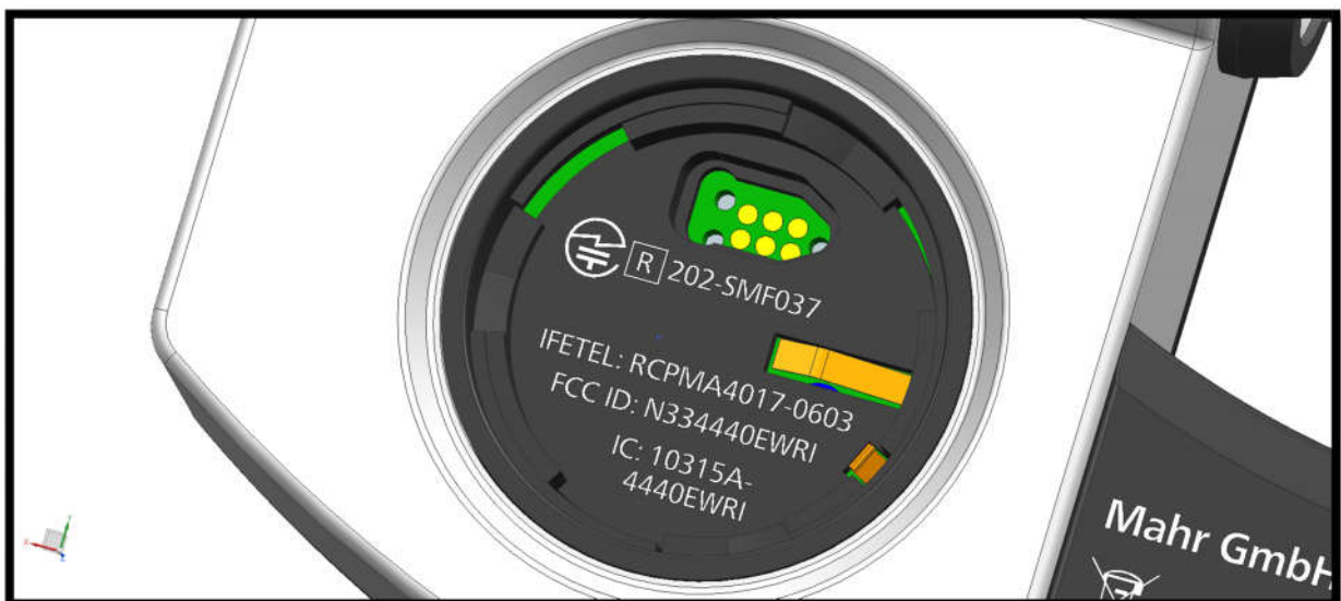
Abbildung 4: Micrometer 40EWri (Certification Numbers up-to-date)
