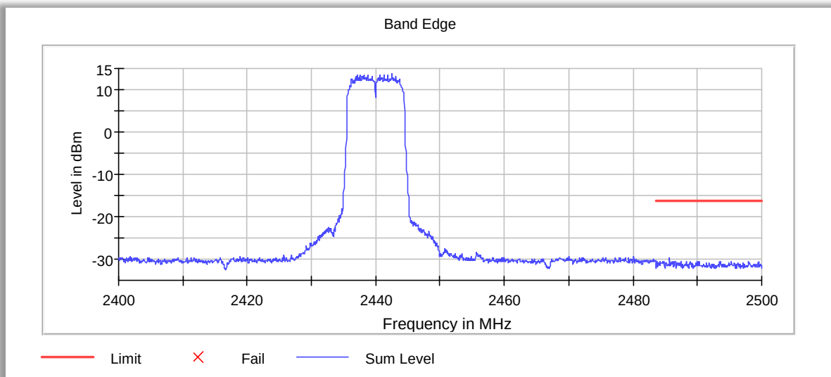
Upper Band Edge 2483.5MHz
