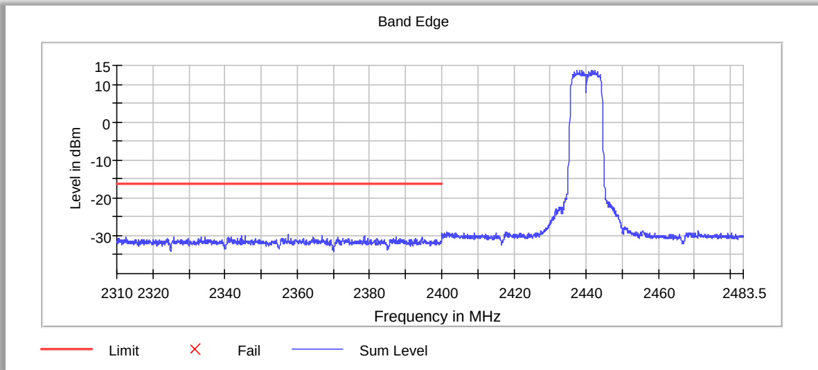
Low Band Edge 2400MHz
