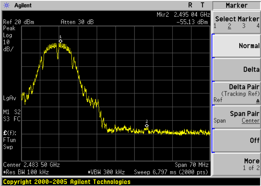
802.11b-CH11
