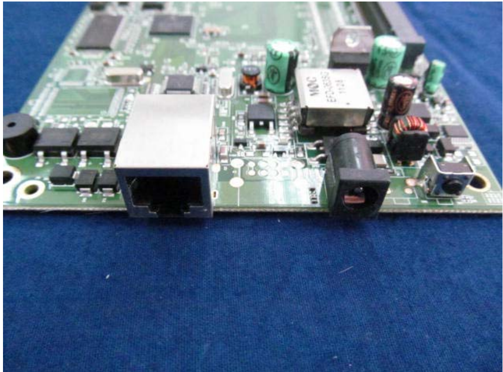
(8) EUT Photo
