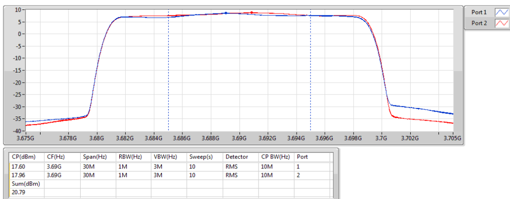
Band 48_LTE_20MHz_Nss1,QPSK_2TX 3690MHz_QPSK_RB 100,#RB 0
