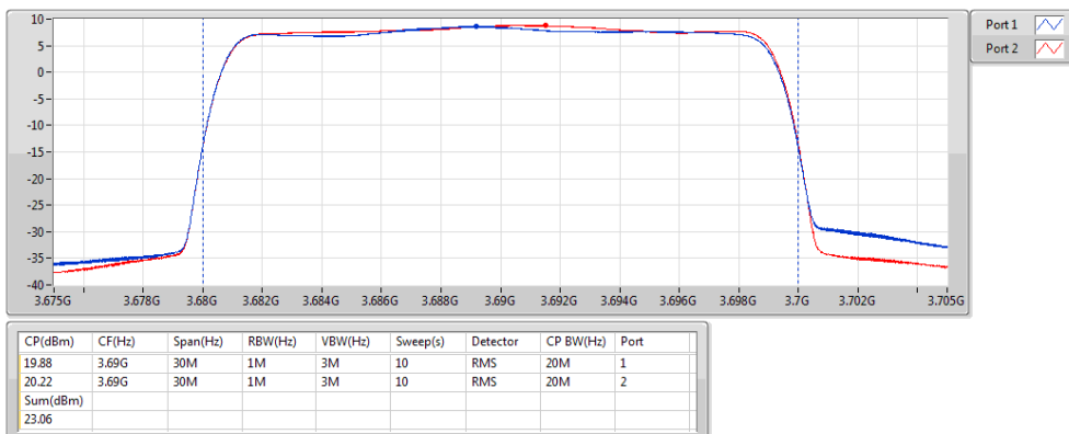
Band 48_LTE_20MHz_Nss1,QPSK_2TX 3690MHz_QPSK_RB 100,#RB 0
