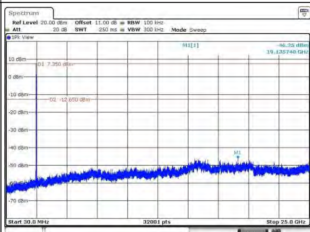
Tx 2480MHz / 30MHz~25GHz (down 20dBc)
