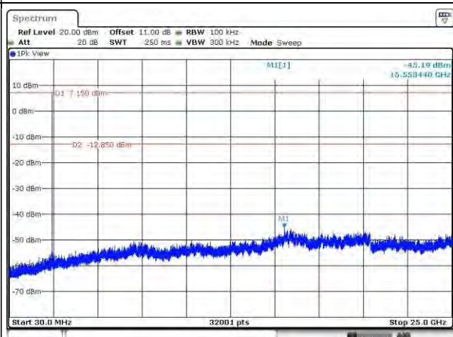
Tx 2440MHz / 30MHz~25GHz (down 20dBc)
