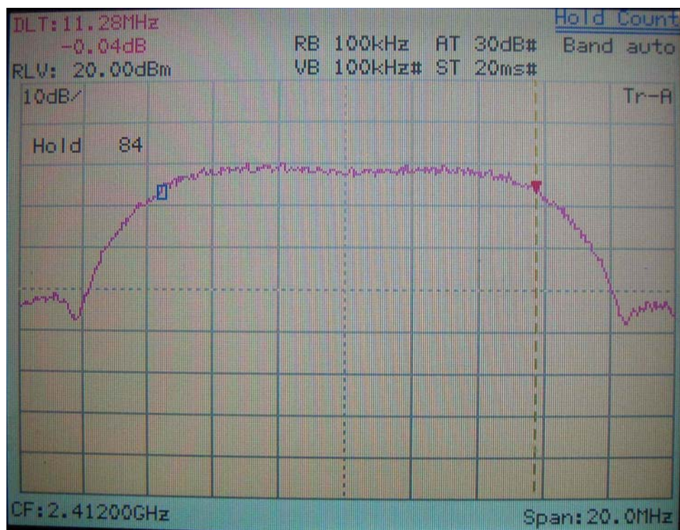
IEEE 802.11b
