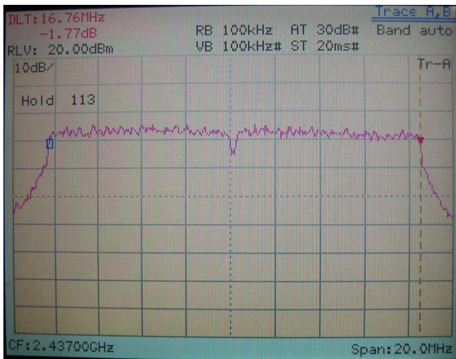
IEEE 802.11g
