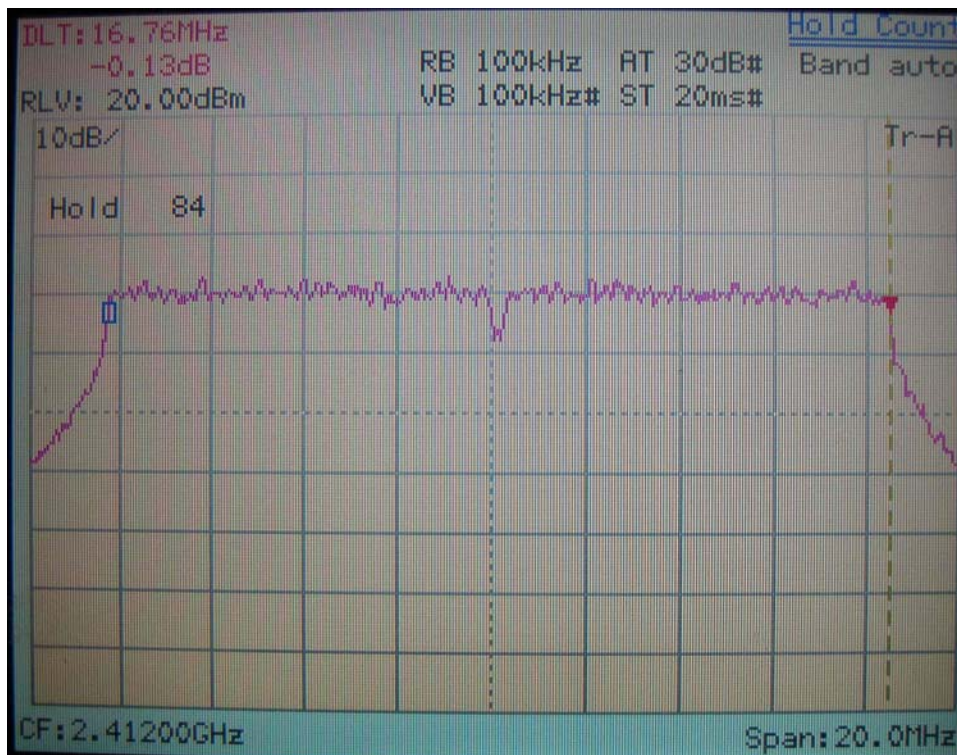
IEEE 802.11g
