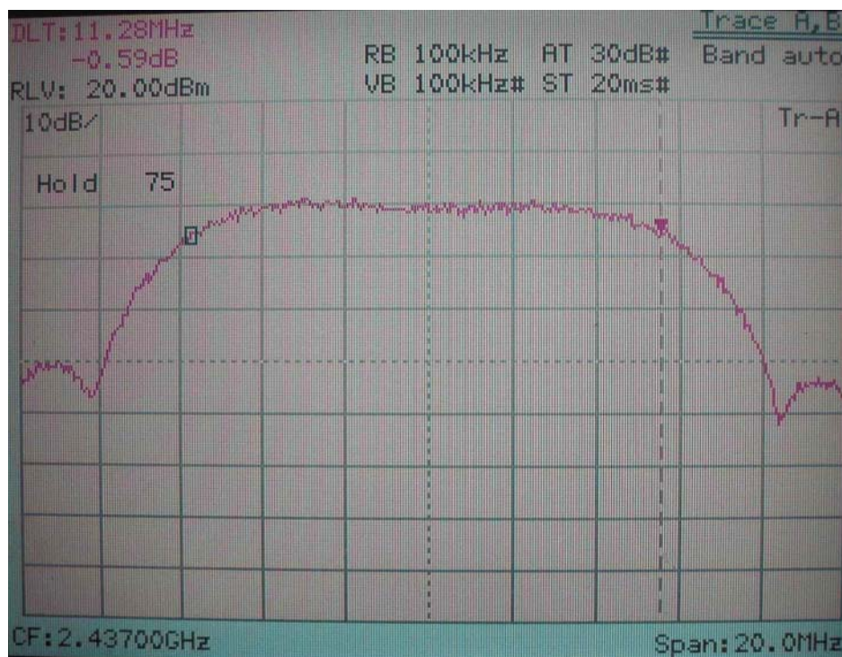
IEEE 802.11b
